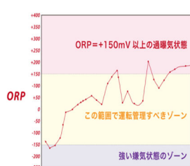
【ORPの運転管理範囲】
