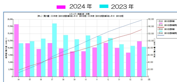
【曝気槽電力消費比較】
